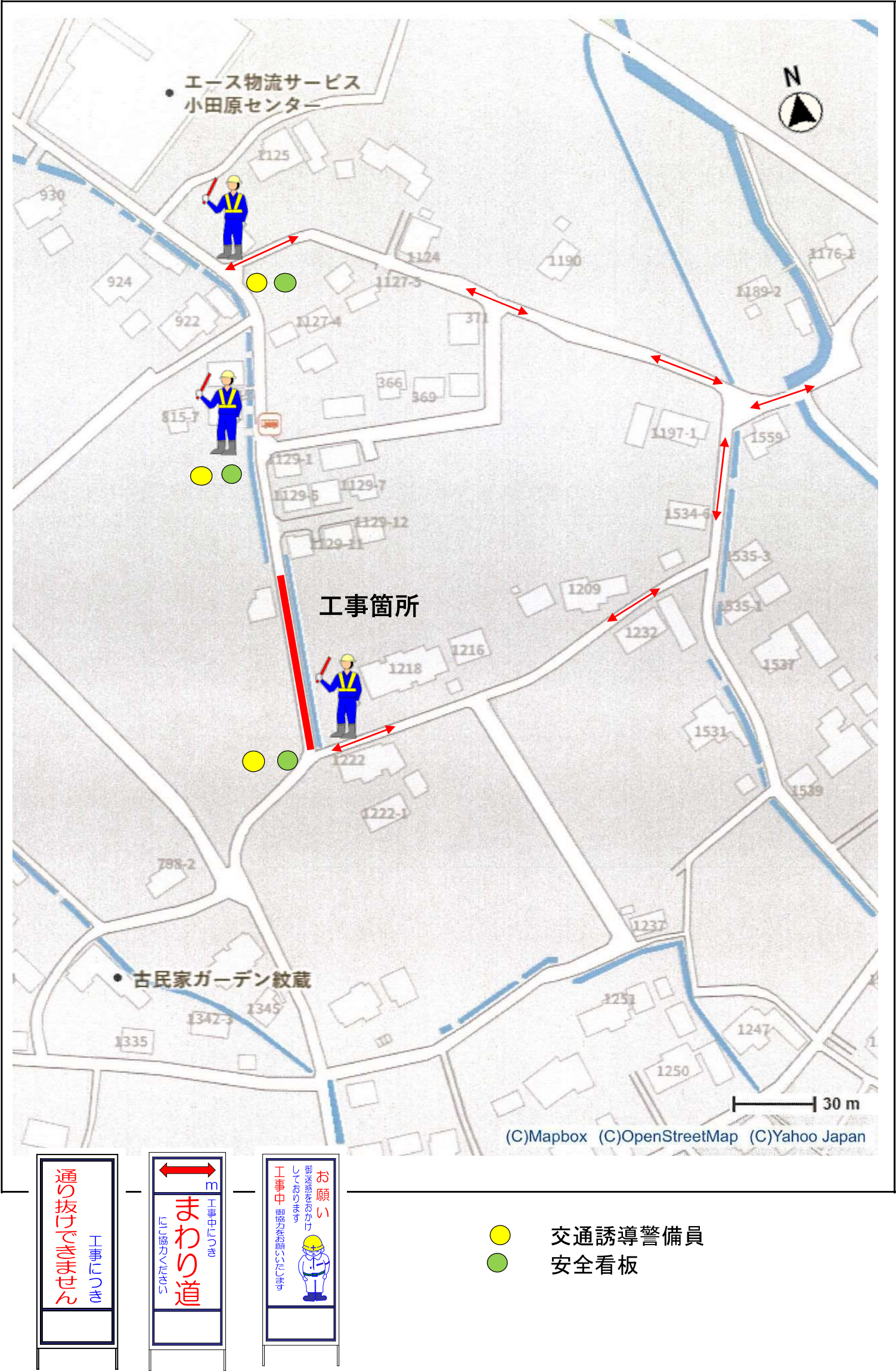
迂回路・交通誘導警備員配置図
