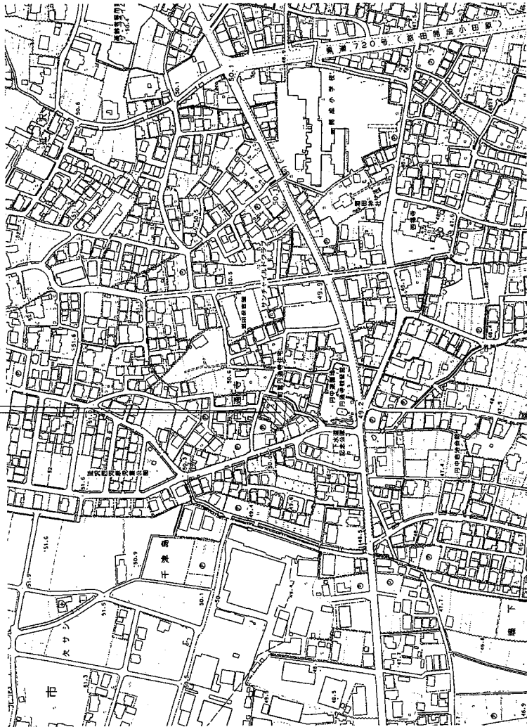
付近星図 S=1:N
